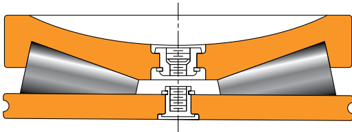
Fig. 23. TTHDFLSV.
